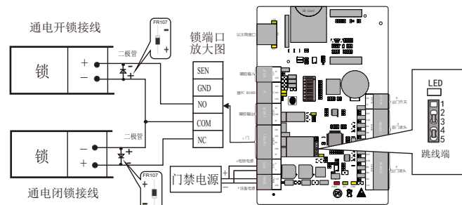
电锁与控制器共用电源“湿模式”接线图
