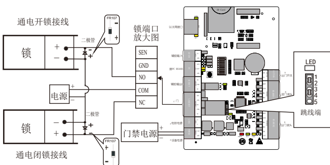
电锁单独供电“干模式”接线图
