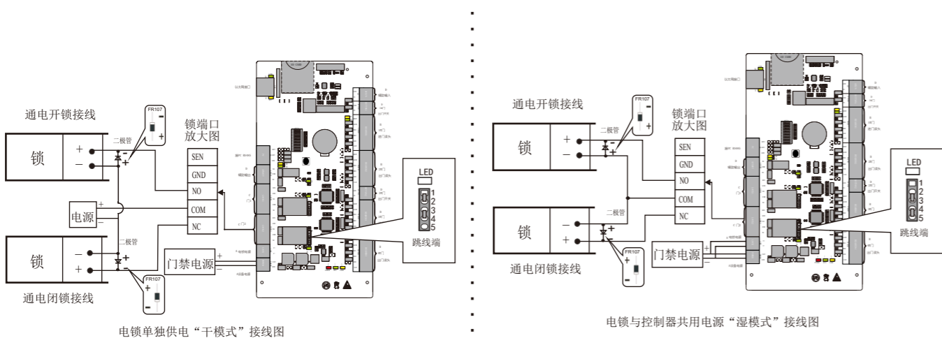
电锁单独供电“干模式”接线图
