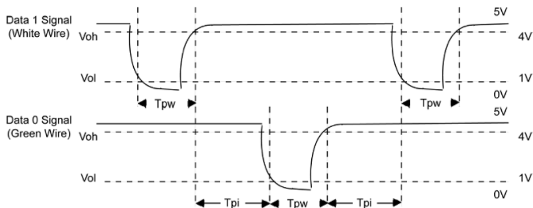
图一 时序图
